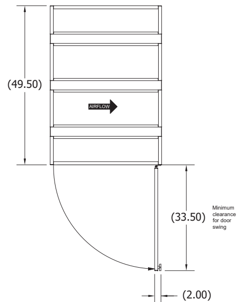
AUTOCLEAN® 8000 & F72C Odor Control Module
